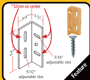
Nylon Kolbe Korner
